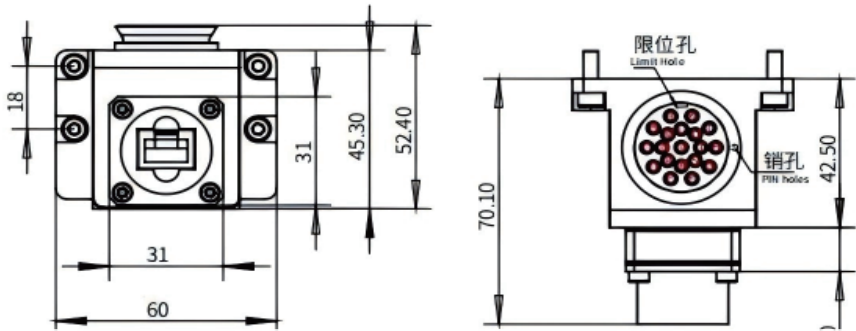
机器人侧模块 Robotside module
