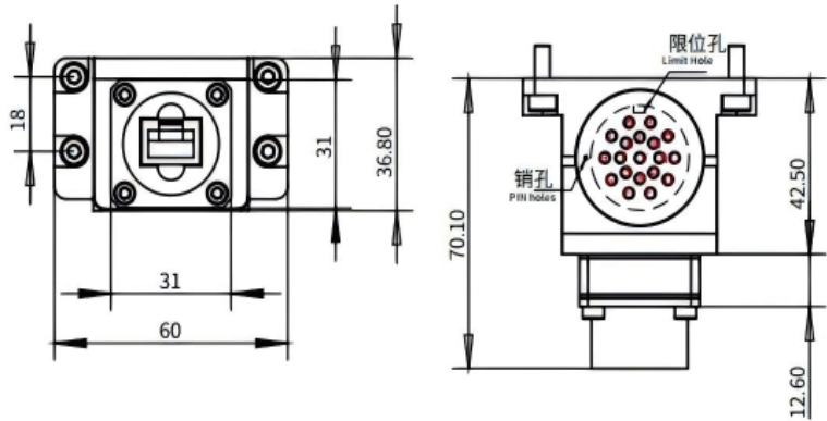
夹具侧模块 Gripperside module
